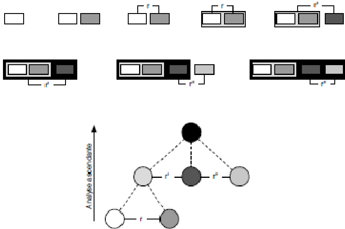
FIG. 5.19 – Analyse ascendante
